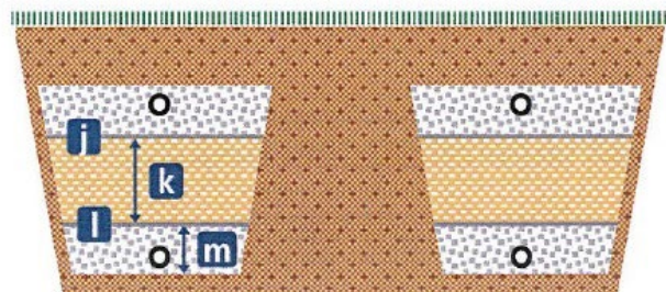
Alt 2: Infiltrationsrör och dräneringsrör i rörgravar
