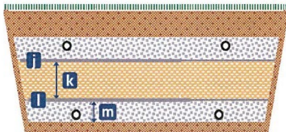
Alt 1: Infiltrationsrör och dräneringsrör i hel bädd
